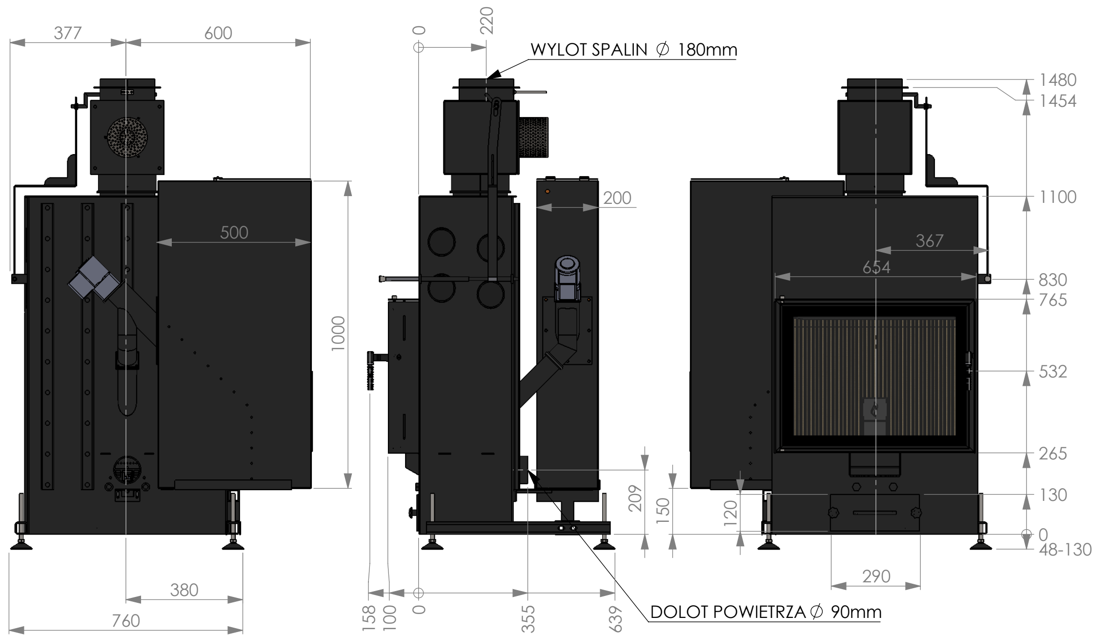
WYMIARY - LOUIS AIR 10kW
