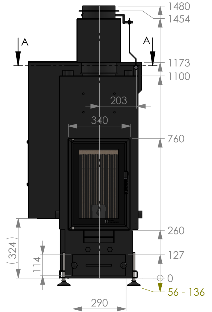
WYMIARY - FELIX AQUA 13 kW
