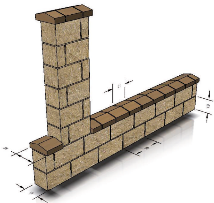
Przęsło ze słupkiem 39 x 19
