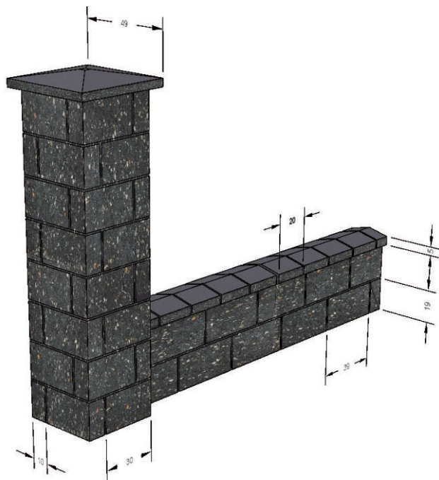
Przęsło ze słupkiem 39 x 39
